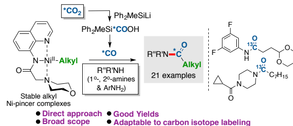
Figur 2: En tilgang til carbonisotop-mærkning af alifatiske carboxamider, der udnytter kuldioxid.
